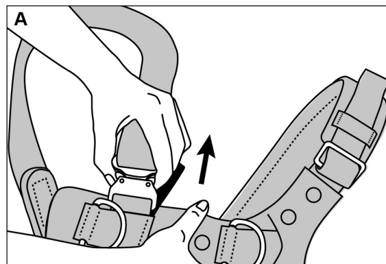
A: Lâcher toutes les boucles et ouvrir la fermeture à pression
